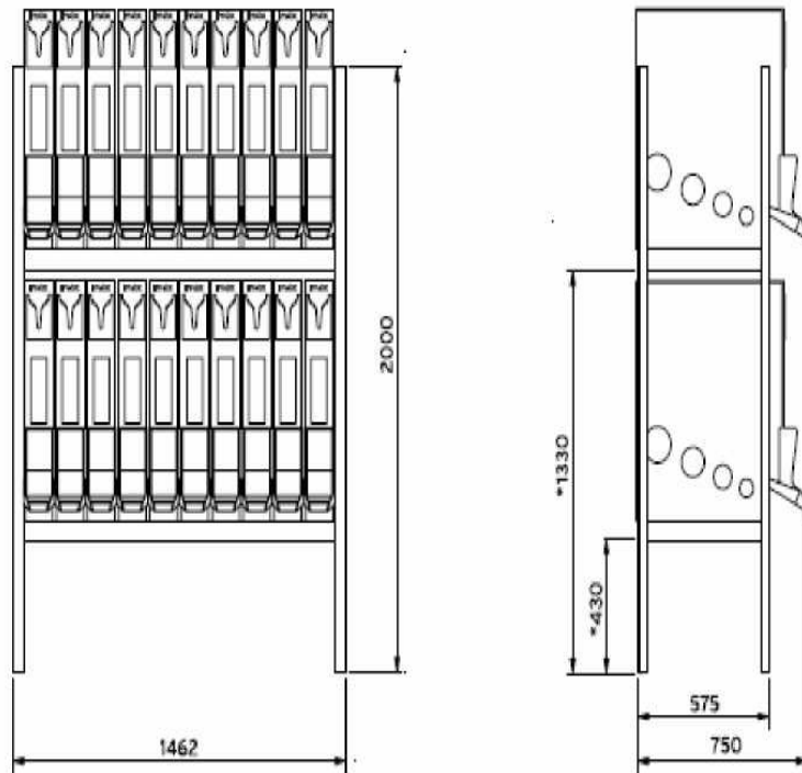
Maße für ein Standregal mit 20 Behältnissen
